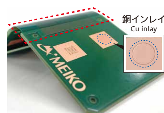
銅インレイ基板と組合せ構造 Structure for Cu inlay and FR4-Flex
