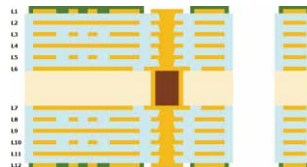
通信モジュール(12層HDI 5-2-5) 基板構造図
