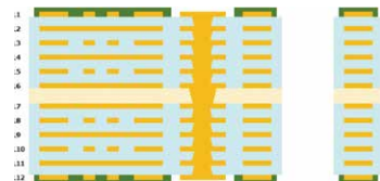
通信モジュール(12層Any layer) 基板構造図
