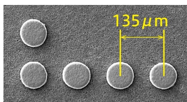
レーザービアピッチ:135μm Laser Via pitch : 135μm
