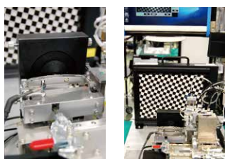
自動フォーカス調整・固定工程
